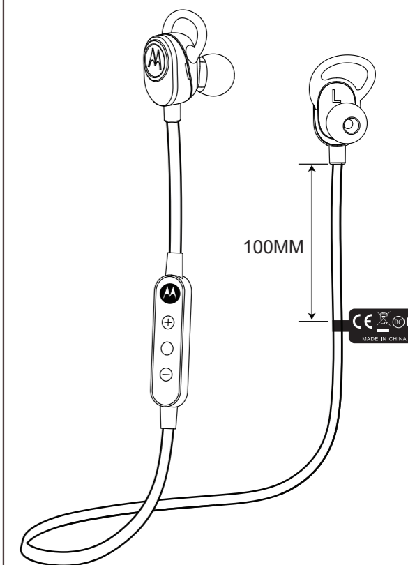
贴附位置
