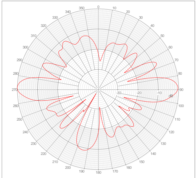
E-Plane 5.85 GHz
