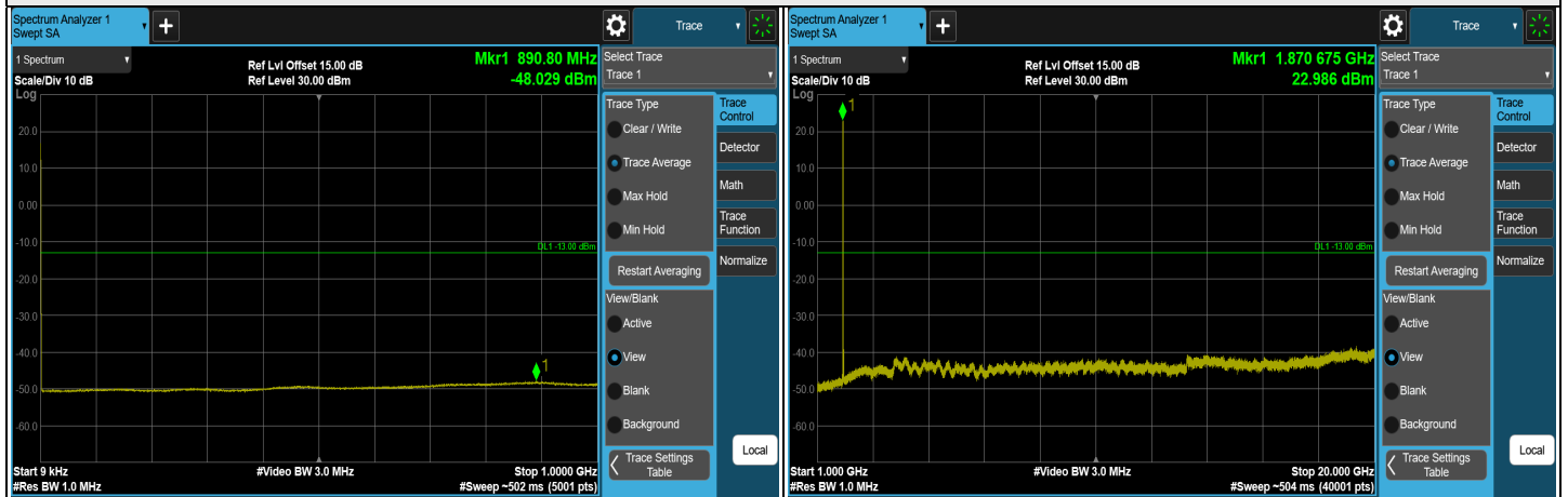
CH 18900 (1880 MHz)
