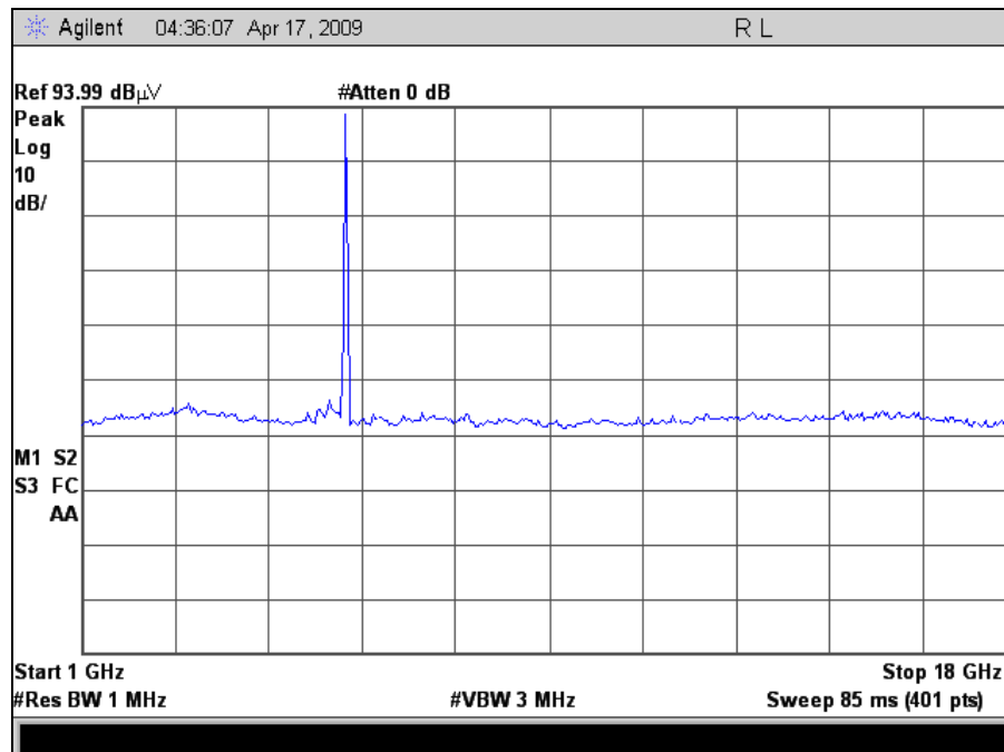
Plot 14. 802.11a Mid Channel (chn 157), 1-18GHz
