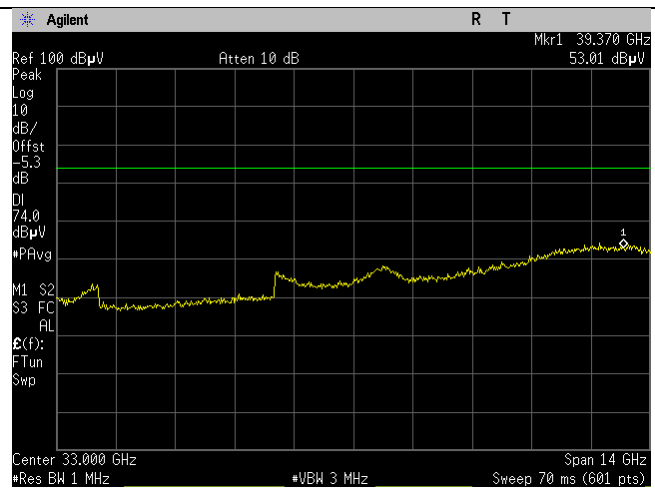
5700MHz_Ch_140_20MHz BW_a-mode_26-40GHz_peak_Ant D
