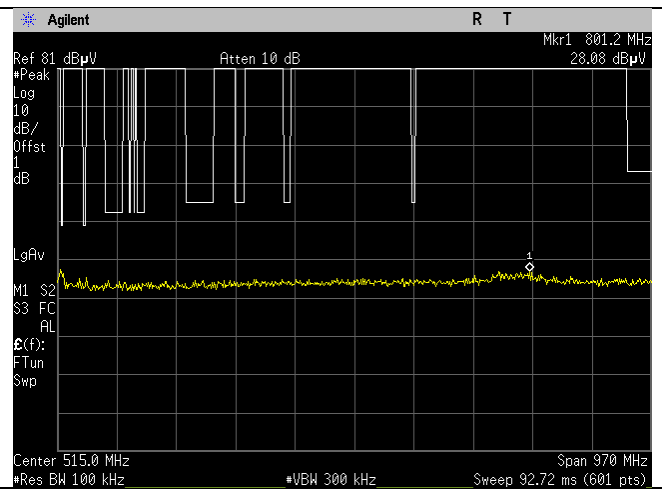
5500MHz_Ch_100_20MHz BWa-mode_30- 1000MHz_Peak_Ant D
