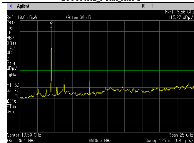
5500MHz_Ch_100_20MHz BW_a-mode_1-26GHz _Peak_Ant C
