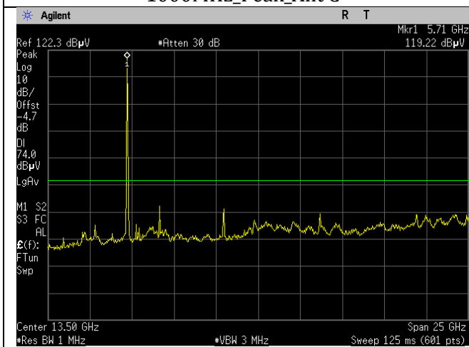
5720MHz_Ch_144_20MHz BW_a-mode_1-26GHz_Peak_Ant C
