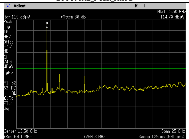
5500MHz_Ch_100_20MHz BW_a-mode_1-26GHz _Peak_Ant D
