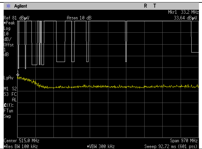
5600MHz_Ch_120_20MHz BWa-mode_30- 1000MHz_Peak_Ant D
