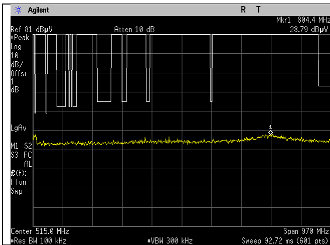
5600MHz_Ch_120_20MHz BWa-mode_30- 1000MHz_Peak_Ant C
