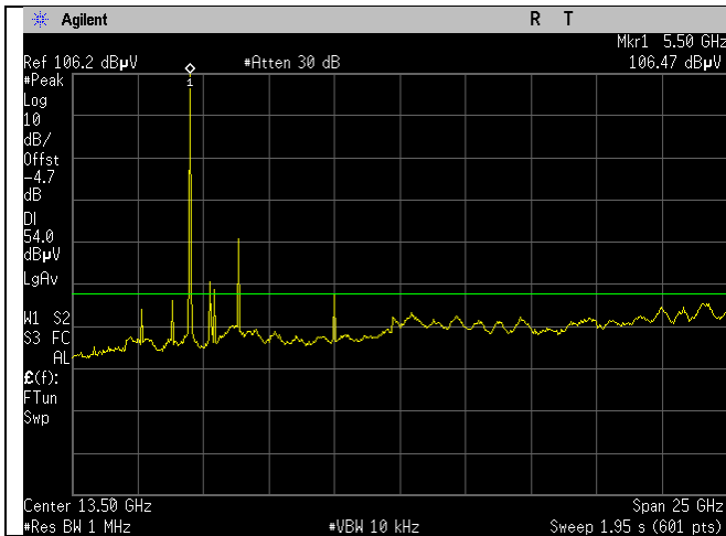
5500MHz_Ch_100_20MHz BW_a-mode_1-26GHz Avg_Ant C
