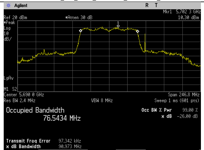
5690MHz_Ch_138_80MHz_ac-mode_Ant B
