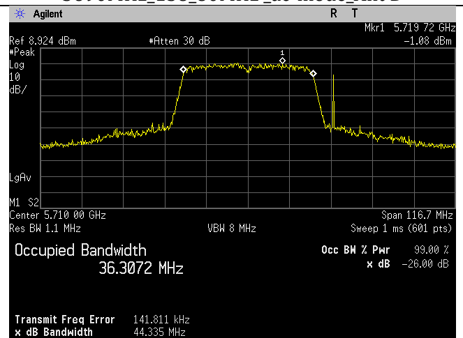
5710MHz_142_40MHz_n-mode_Ant D
