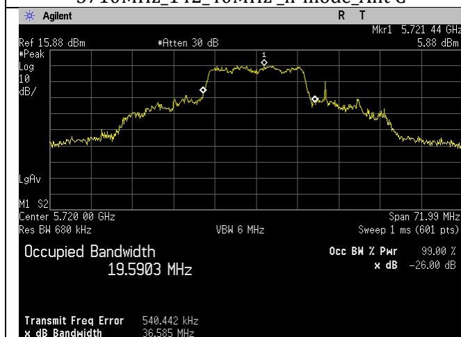
5720MHz_144_20MHz_a-mode_Ant C
