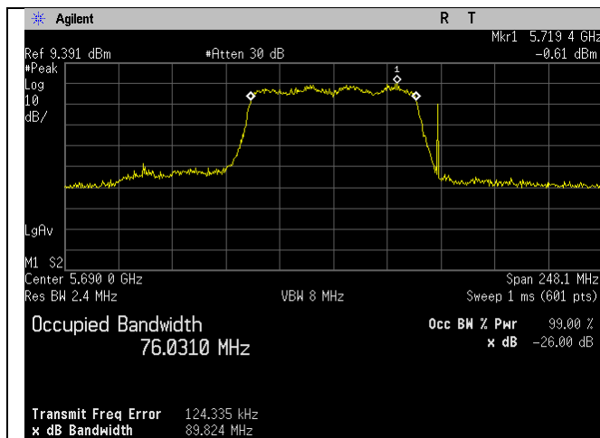
5690MHz_138_80MHz_ac-mode_Ant C
