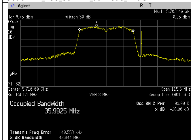
5710MHz_142_40MHz_n-mode_Ant C
