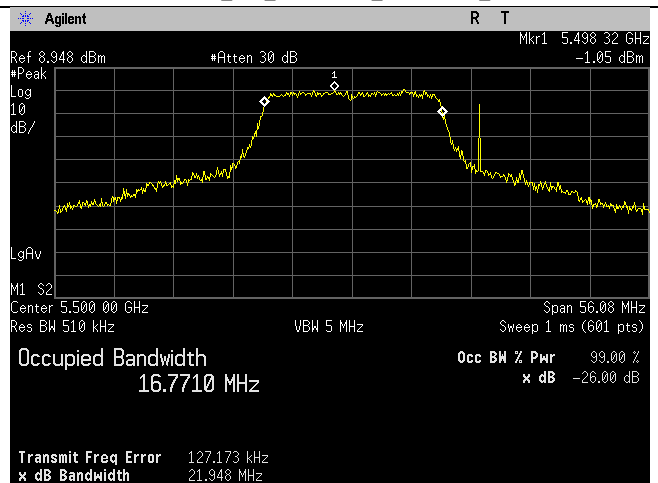
5500MHz_100_20MHz_a-mode_Ant D
