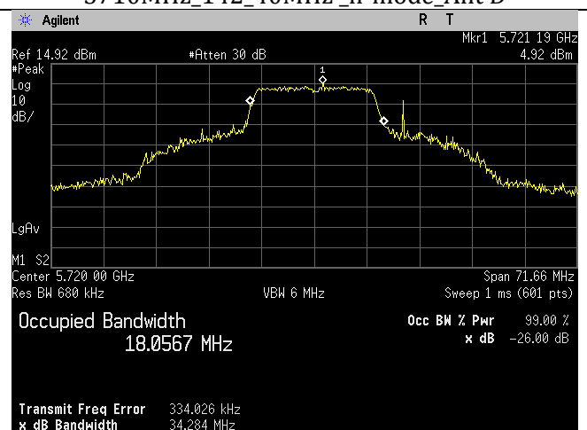
5720MHz_144_20MHz_a-mode_Ant D
