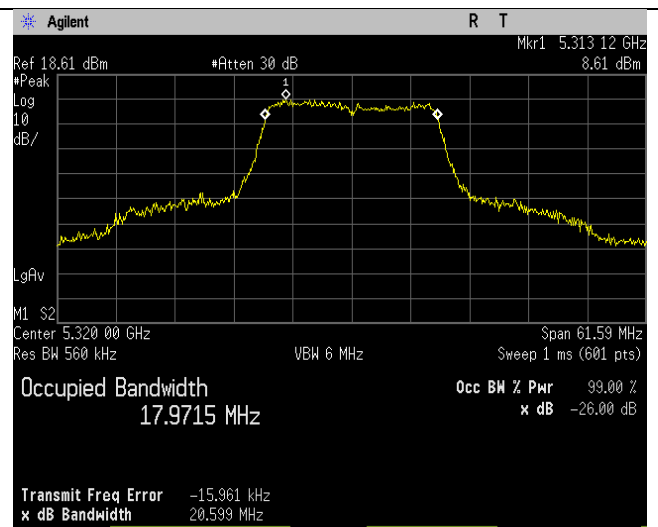
5320MHz_64_20MHz_n-mode_Ant D
