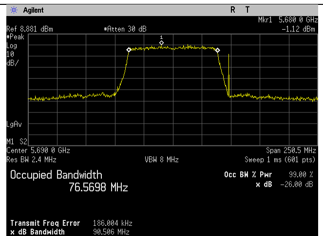
5690MHz_138_80MHz_ac-mode_Ant D
