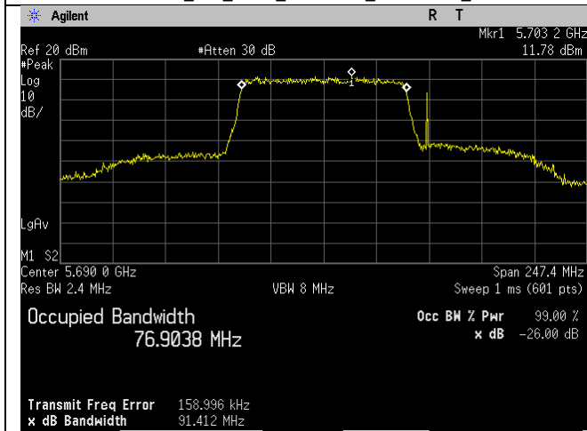
5690MHz_Ch_138_80MHz_ac-mode_Ant A
