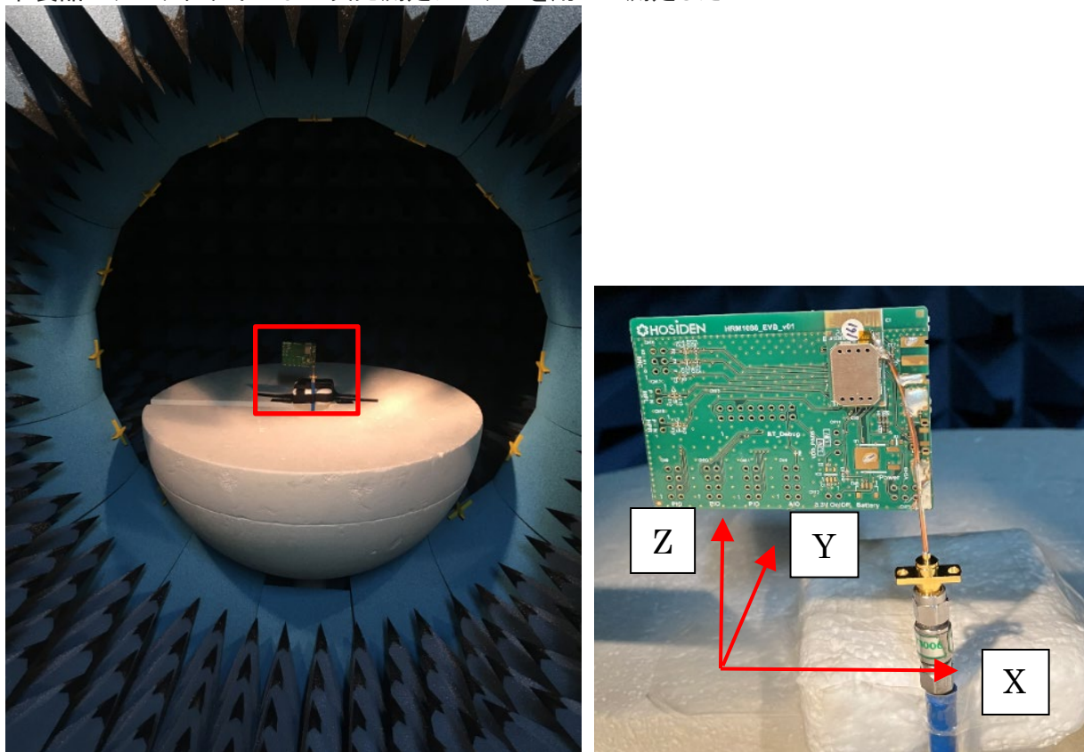
Figure 2: Antenna gain measurement /アンテナゲインの測定
