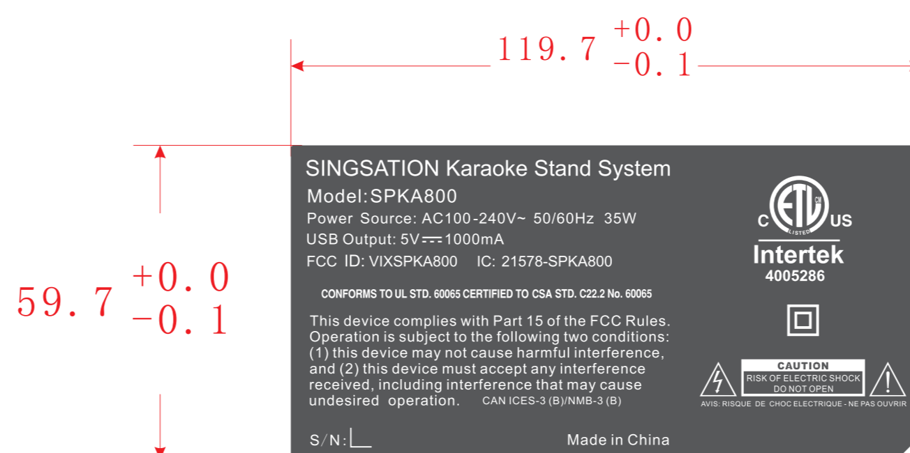
标签贴纸尺寸图
