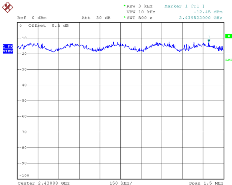
PLOT T6B : 802.11g, Middle Channel, Antenna 0 (Con 1)
