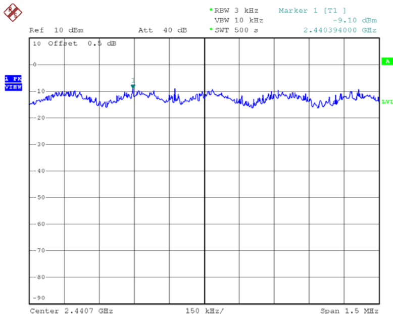
PLOT E6B : 802.11g, Middle Channel, Antenna 1 (Con 2)
