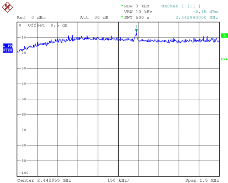
PLOT T5B : 802.11b, Middle Channel, Antenna 0 (Con 1)
