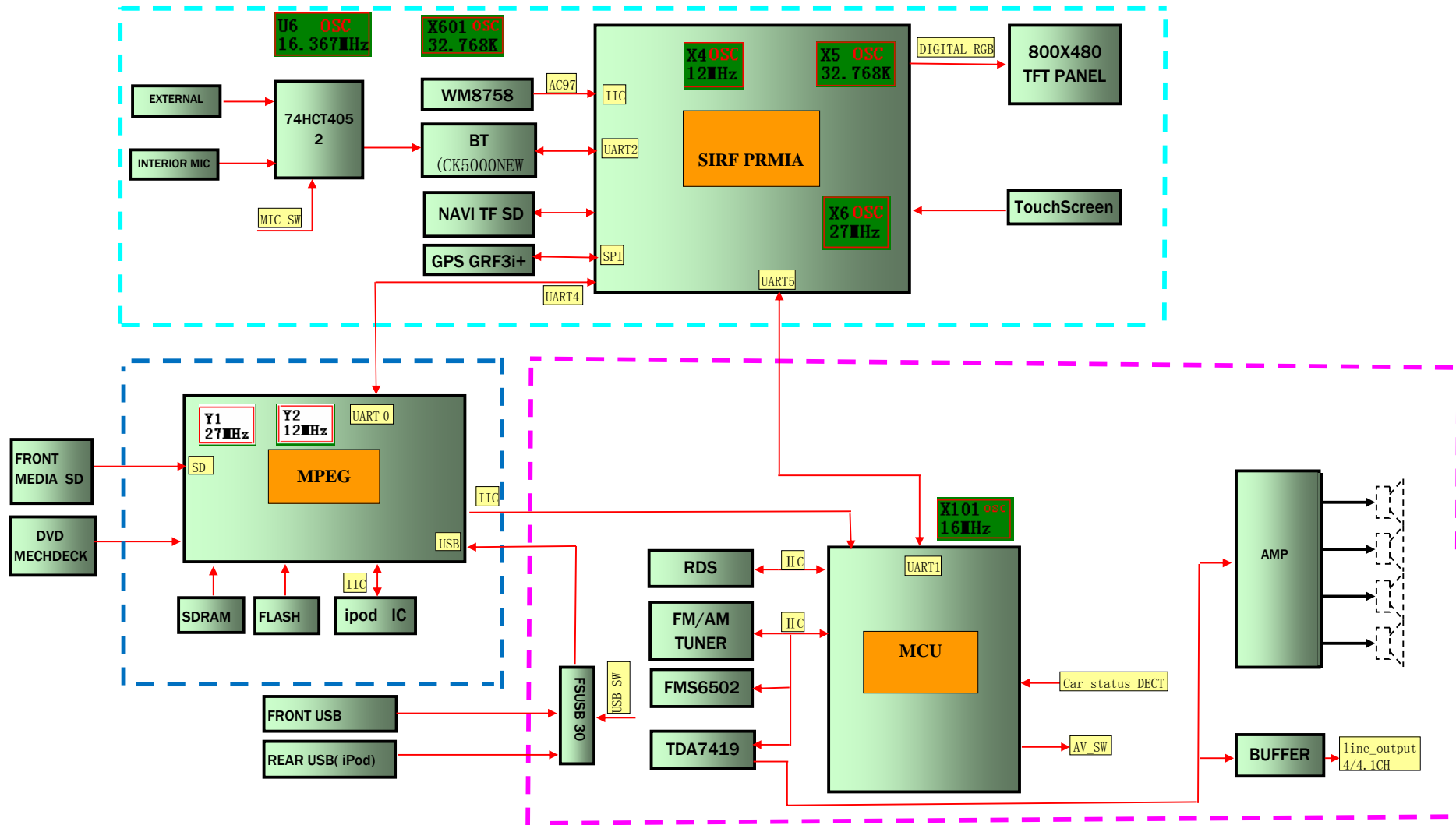
CE6904 ARM11 PRIMA系统框图 V00
