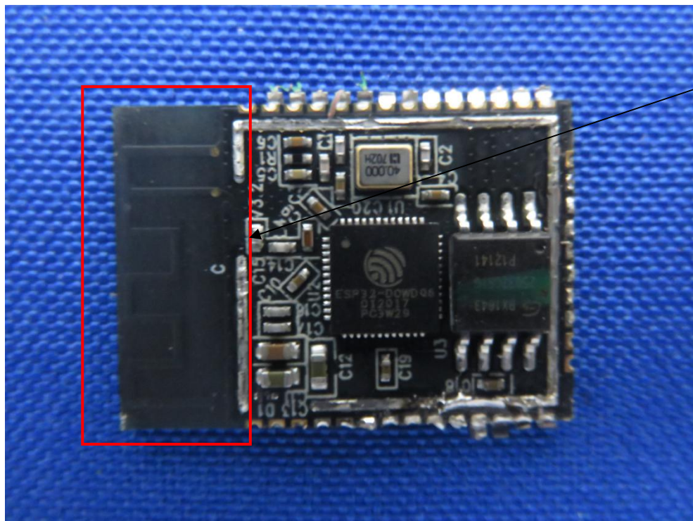
BT&WiFi Antenna
