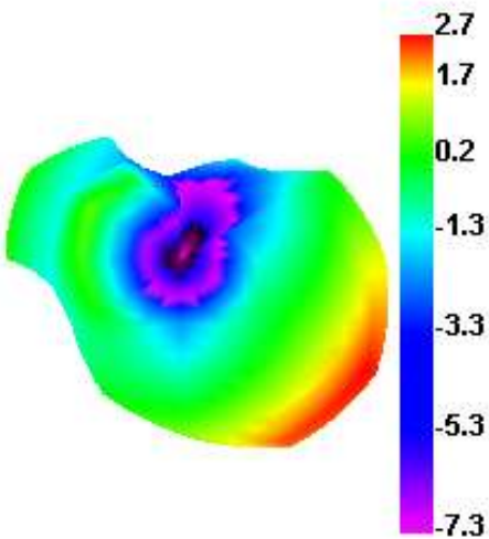
2450.000MHz
