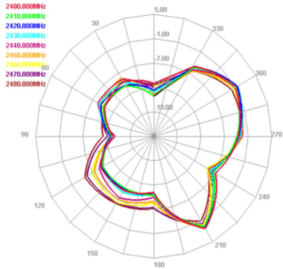
2480.000MHz
