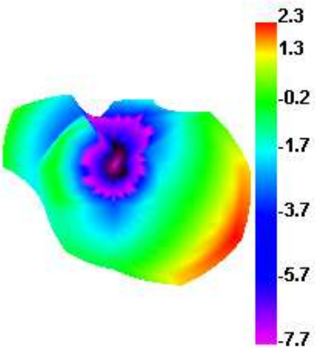
2480.000MHz
