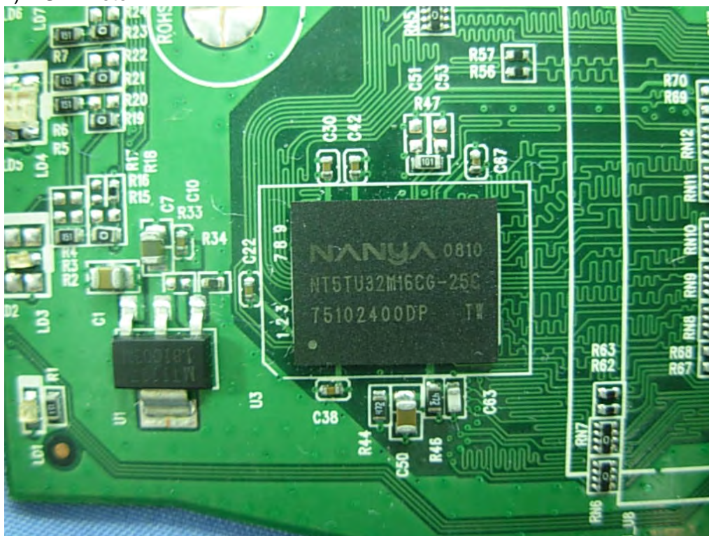
(17) EUT Photo
