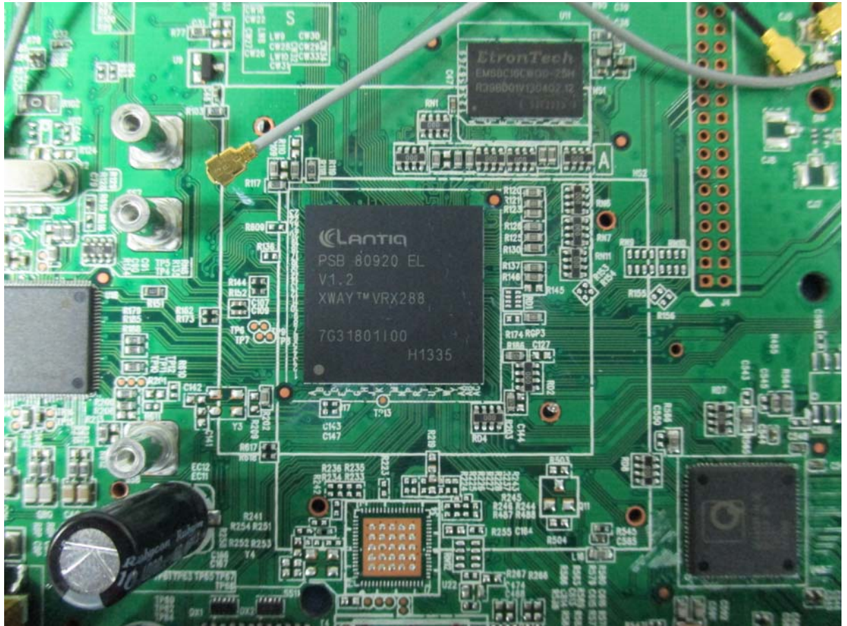
(18) EUT Photo (CPU)
