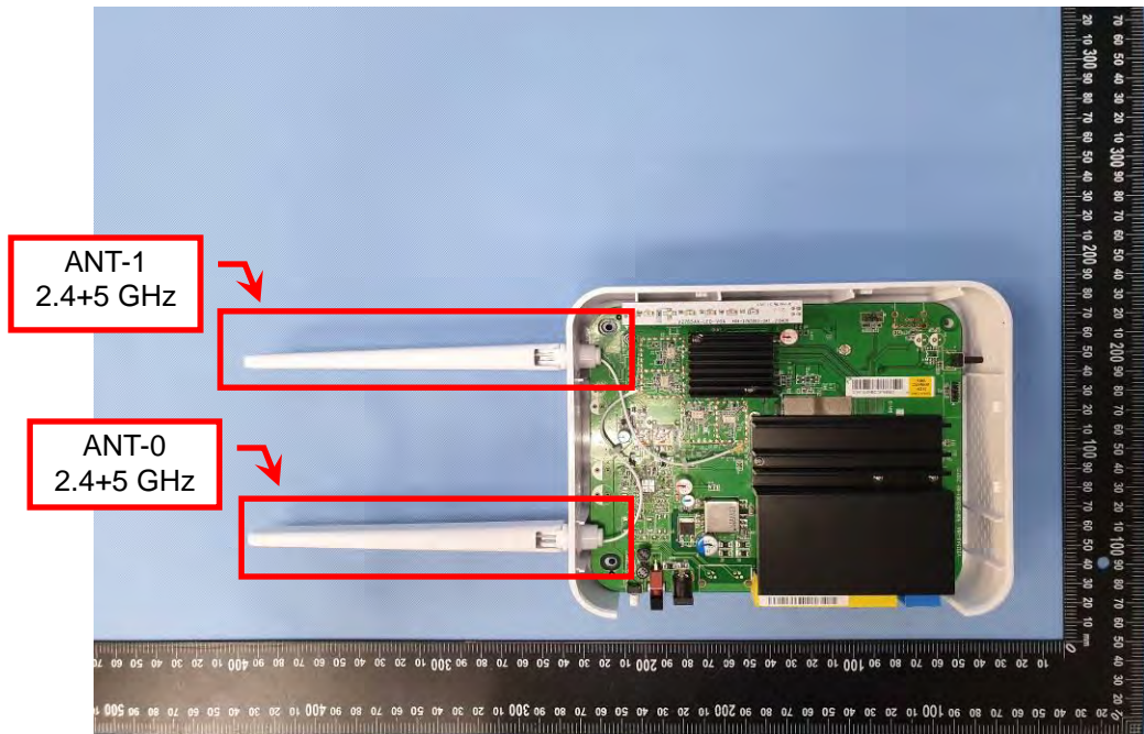
EUT Photo (2)
