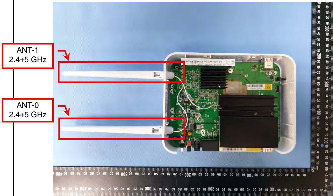
EUT Photo (2)
