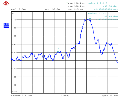
Port 2, 2400 MHz Band Edge
