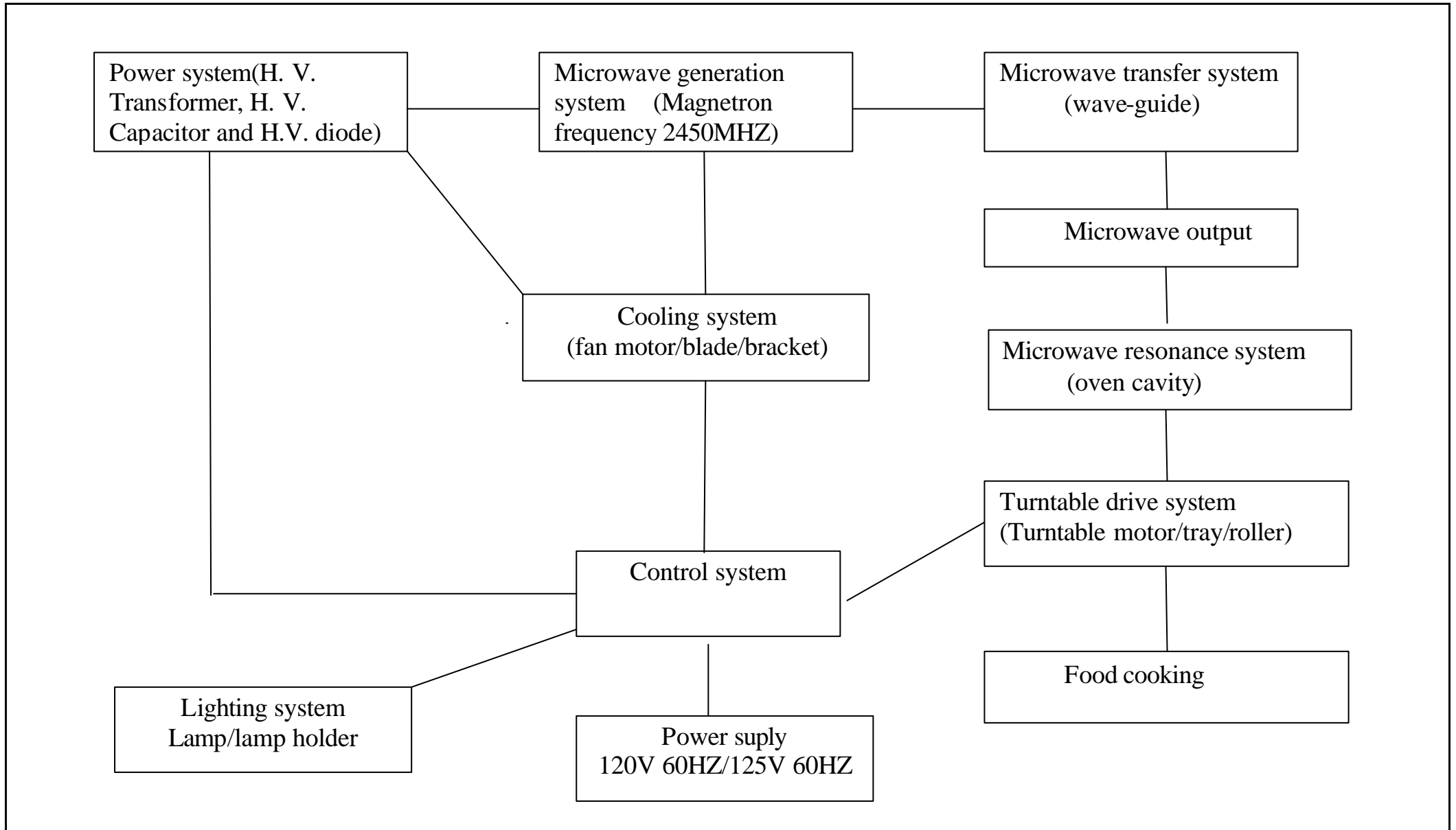
XM942KYY 产品方框图
