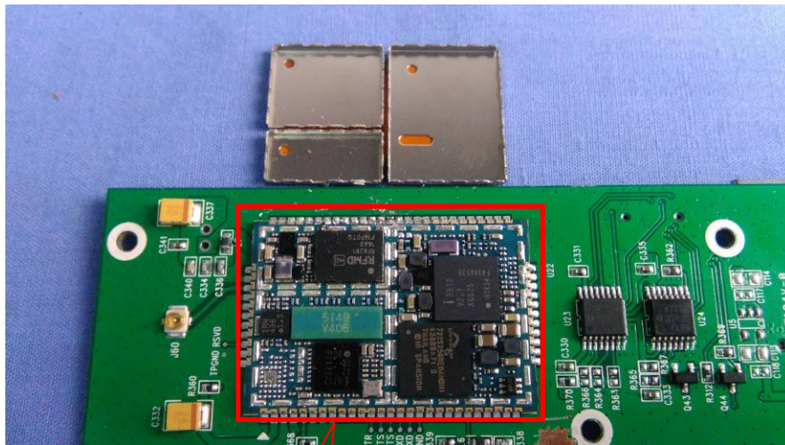
RF Module
