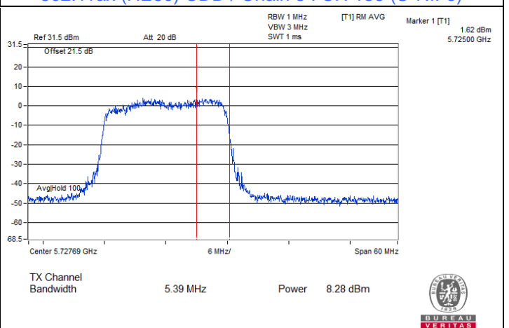
802.11ax (HE20) CDD_RU242 / Chain 0 : CH 144 (U-NII-3)
