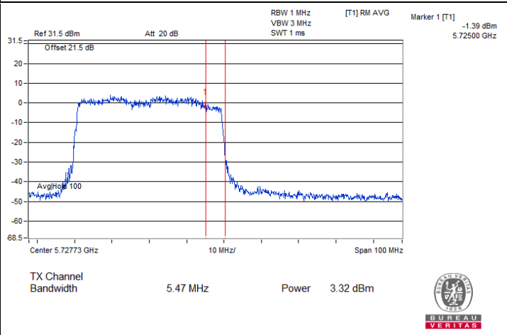
802.11ax (HE40) CDD_RU484 / Chain 2 : CH 142 (U-NII-3)
