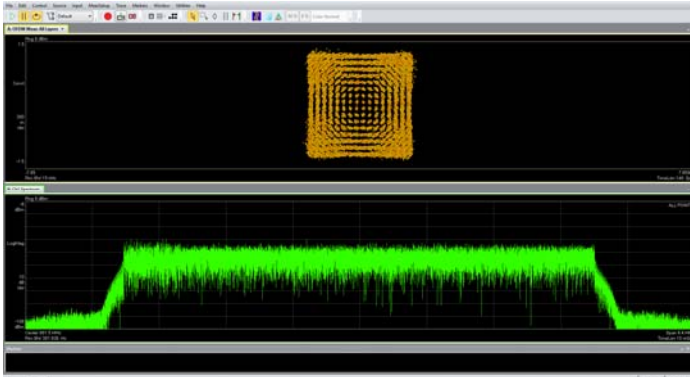
256QAM (TM3.1a) 881.5MHz
