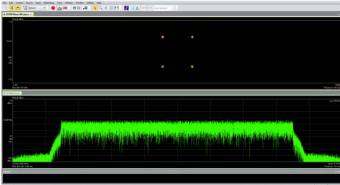
QPSK (TM1.1), 889MHz
