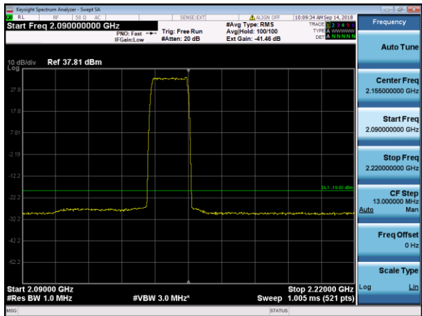
LTE15 Top+NB IoT GB (Upper) 2090MHz-2220MHz
