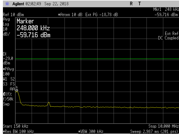
LTE10 Mid+NB IoT GB (Upper) 0.15MHz – 10MHz
