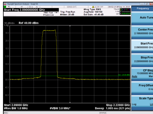
LTE15 Mid+NB IoT GB (Upper) 2090MHz-2220MHz
