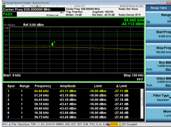
9KHz – 150kHz
