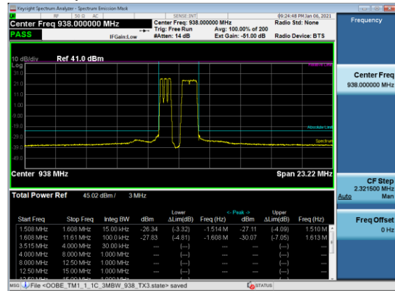
TM 1.1 / QPSK / 938.0MHz / 0.2+0.2+0.2+1.4MBW / TX3
