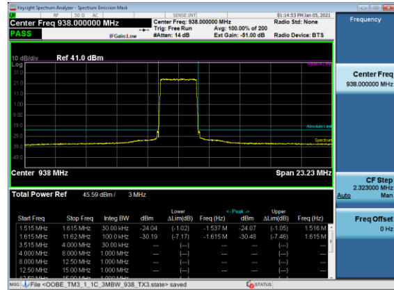
TM 3.1 / 64QAM / 938.0MHz / 3MBW / TX3
