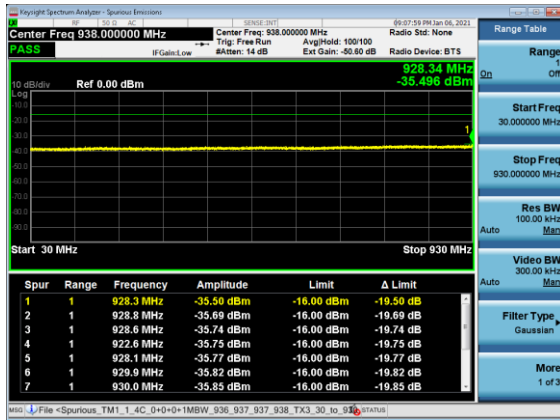
30MHz – 930MHz
