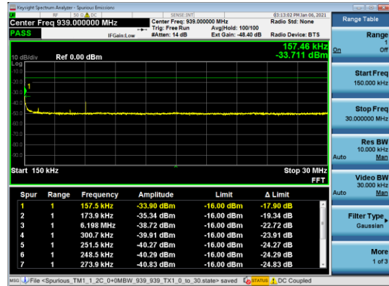
150kHz – 30MHz
