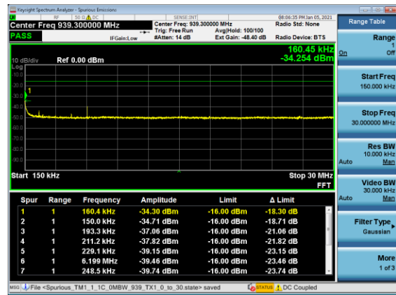
150kHz – 30MHz
