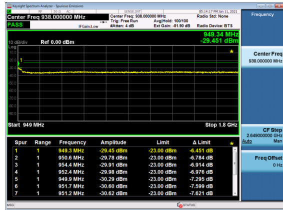
949MHz – 1.8GHz
