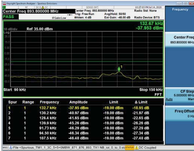
90kHz – 150kHz
