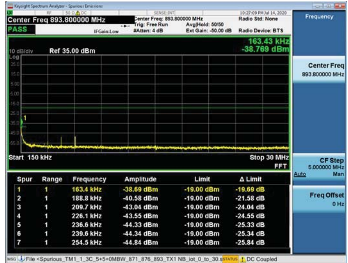
150kHz – 30MHz
