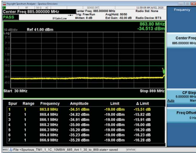
30MHz – 869MHz
