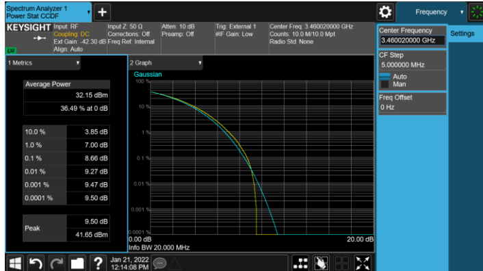
TM 3.1a / 256QAM / 3460MHz / TX15
