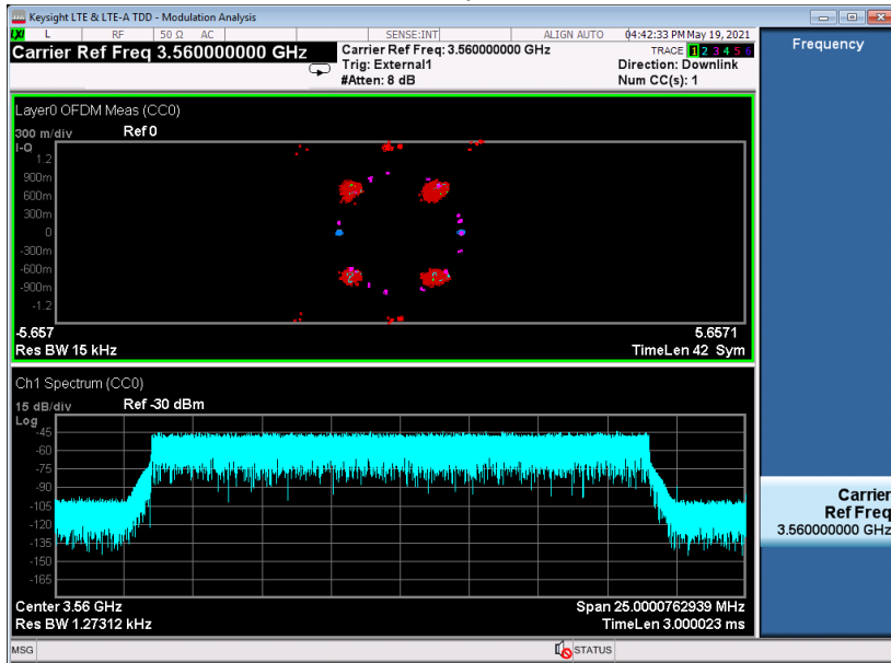
Modulation QPSK TM1.1
