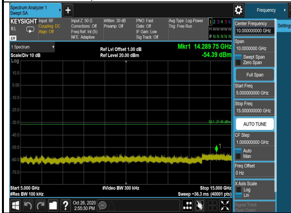
802.11n(HT40),2452MHz,Ant0,Plot 5,5000MHz~15000MHz
