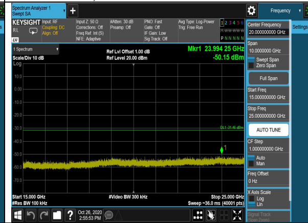
802.11n(HT40),2452MHz,Ant0,Plot 6,15000MHz~25000MHz
