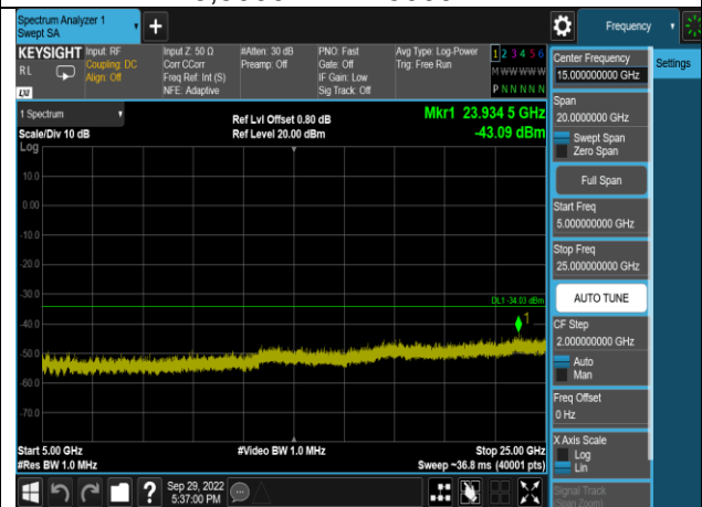
802.11n(HT40),2452MHz,Ant0,Plot 5,5000MHz~25000MHz
