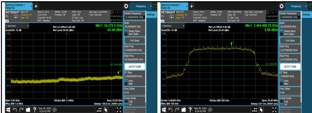
802.11g,2462MHz,Ant0,Plot 2,Band Edge
