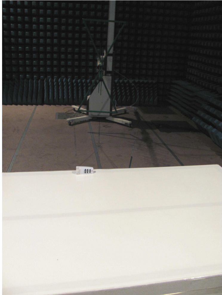
30MHz-1000MHz, Y axis
