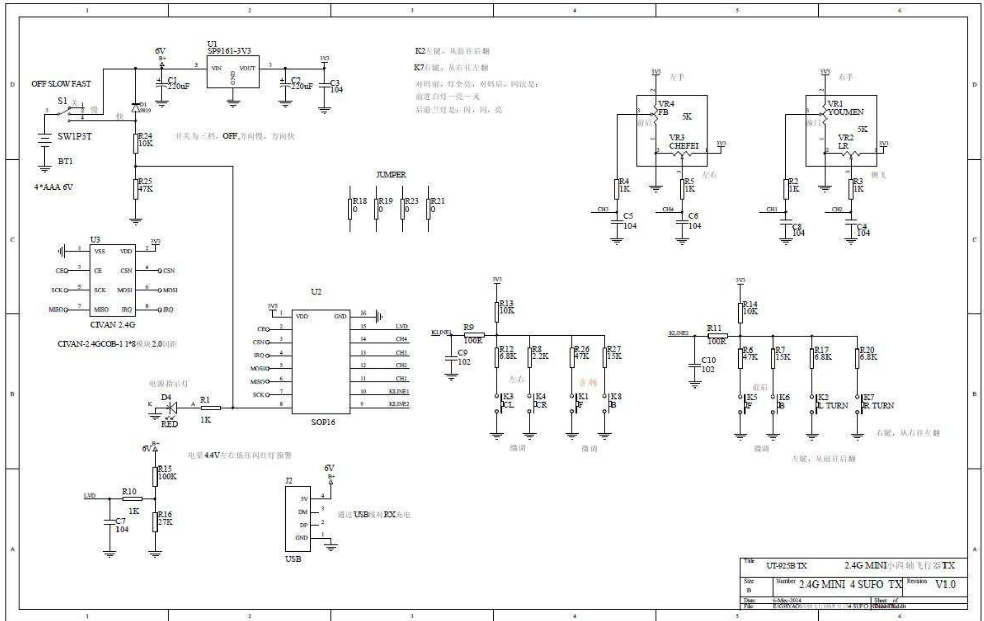
236TX微調自轉電路圖 (1177x759x16M png)
