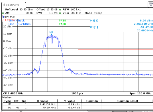
b_2462MHz_Chain 0
