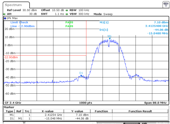
b_2412MHz_Chain 1
