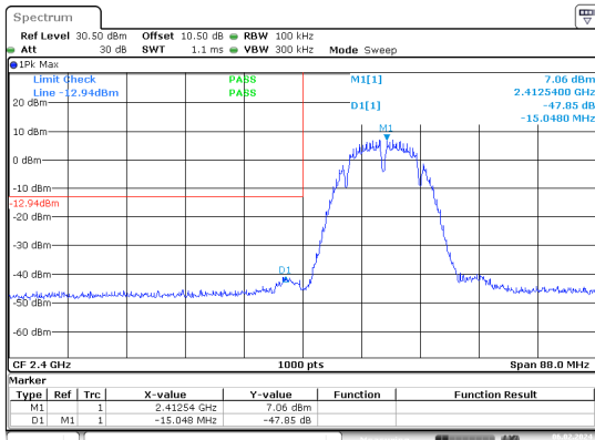
b_2412MHz_Chain 0
