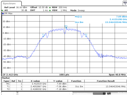
b_2412MHz_Chain 0
