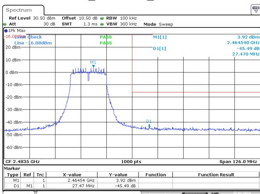
n20_2462MHz_Chain 0
