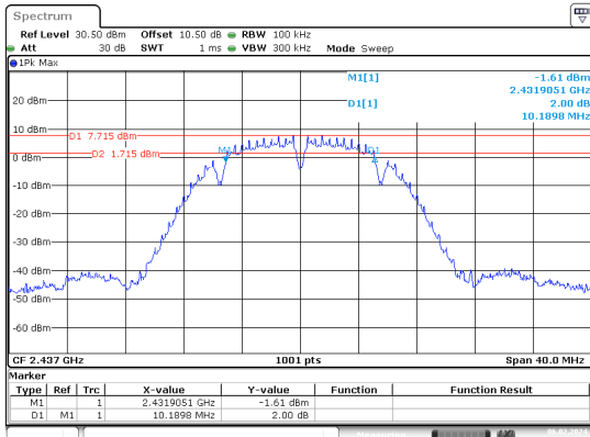
b_2437MHz_Chain 0
