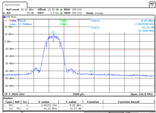
b_2462MHz_Chain 1
