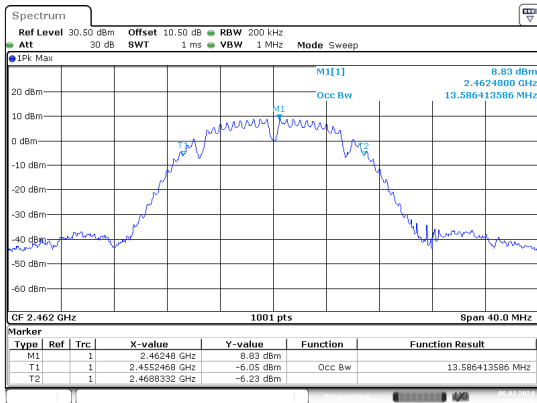
b_2462MHz_Chain 0
