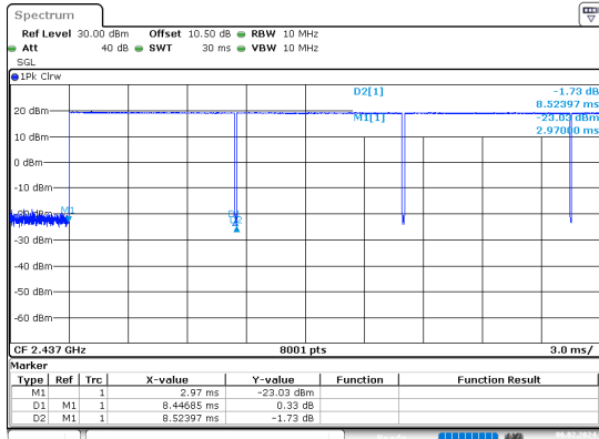
b_2437MHz_Chain 0
