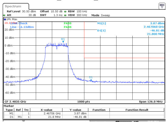
n20_2462MHz_Chain 1
