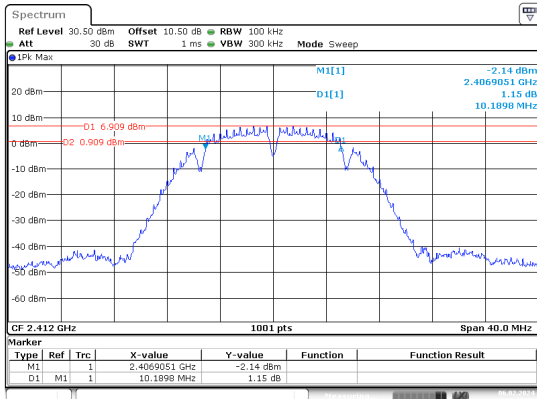
b_2412MHz_Chain 0
