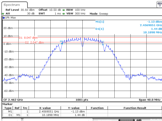
b_2462MHz_Chain 0
