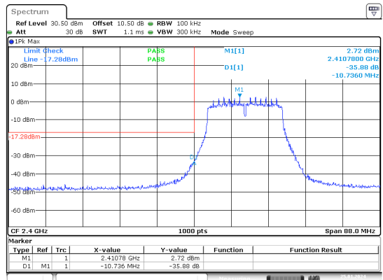
n20_2412MHz_Chain 1
