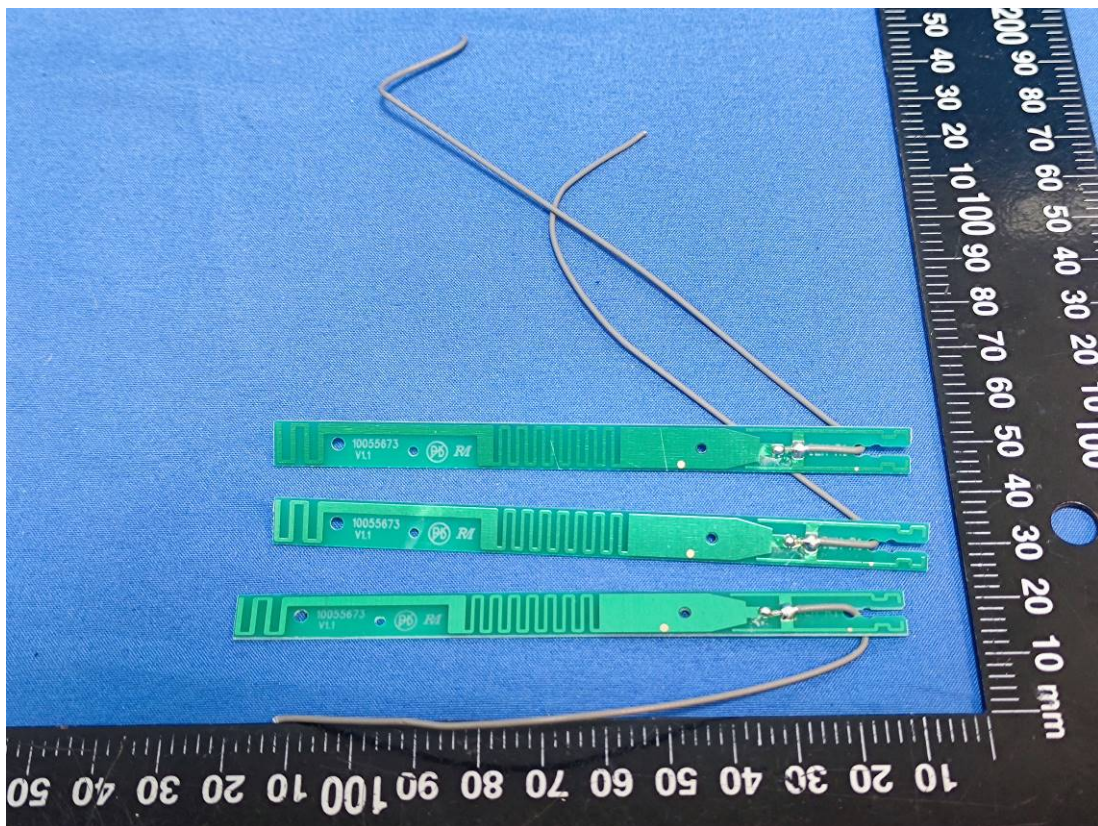
2.4G Antenna
