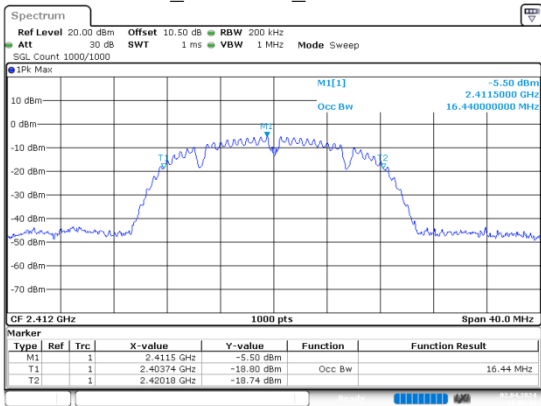
b_2412MHz_Chain 0
