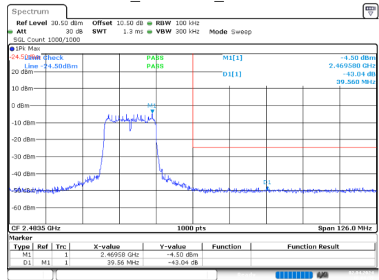
n20_2462MHz_Chain 0
