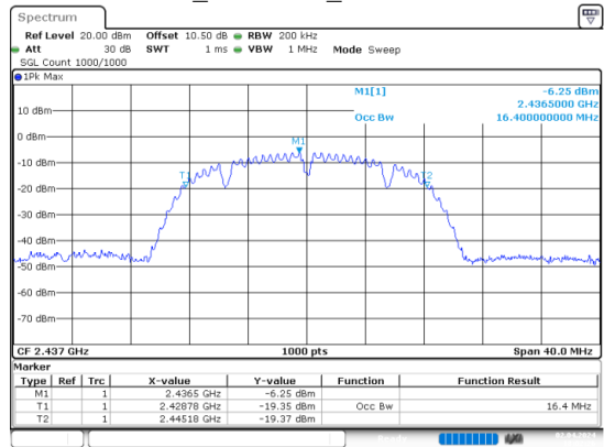
b_2437MHz_Chain 0
