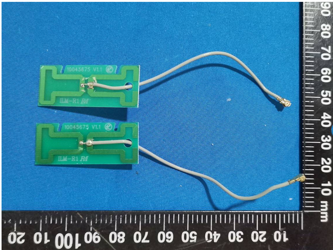
2.4G ANT
