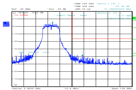
n20_2462MHz_Chain 0
