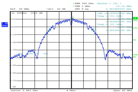
b_2462MHz_Chain 0
