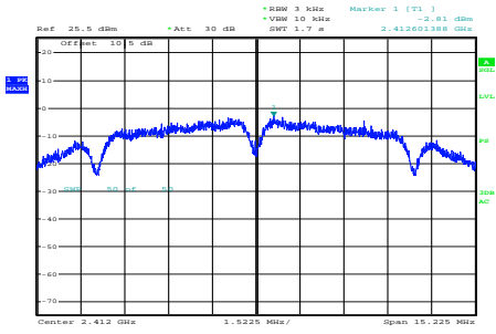
b_2412MHz_Chain 0
