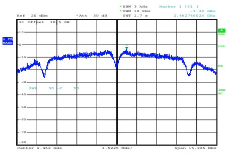
b_2462MHz_Chain 0
