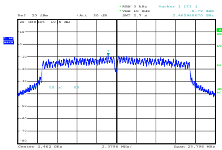
n20_2462MHz_Chain 0
