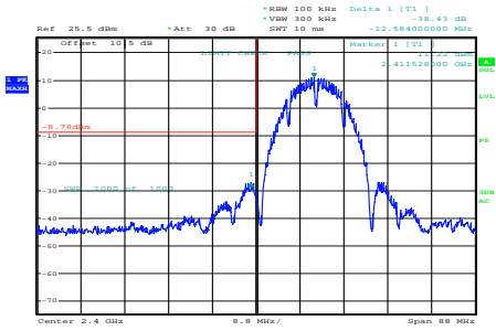
b_2412MHz_Chain 0
