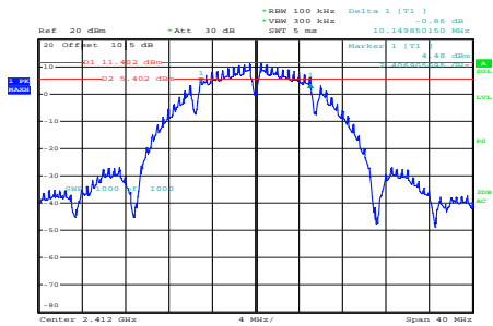
b_2412MHz_Chain 0
