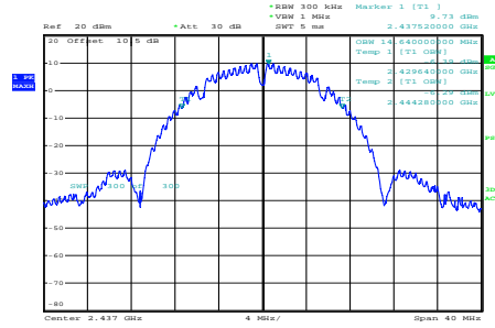
b_2437MHz_Chain 0
