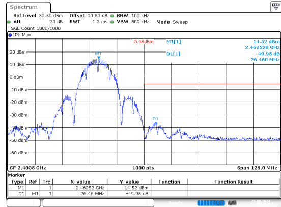
b_2462MHz
