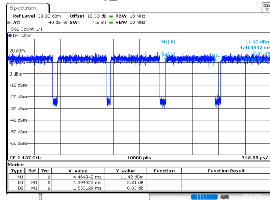
g_2437MHz
