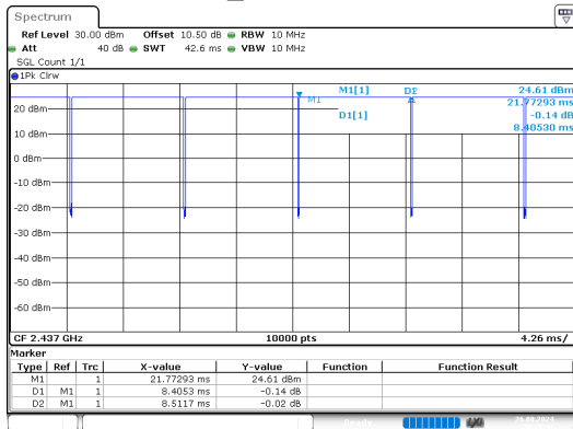
b_2437MHz
