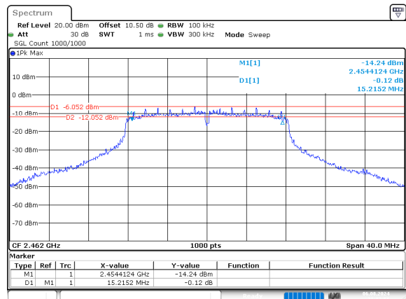
g_2462MHz
