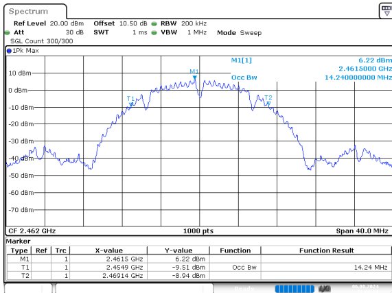
b_2462MHz
