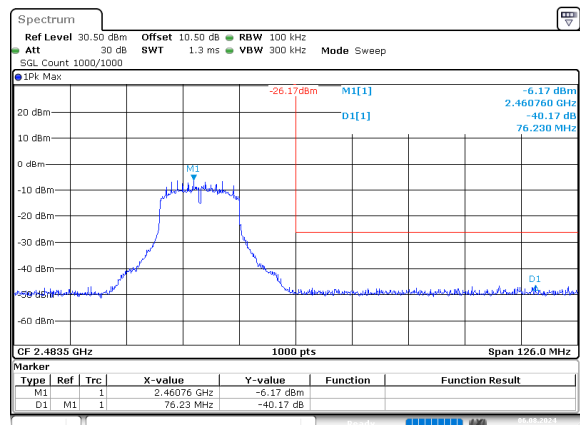
n20_2462MHz
