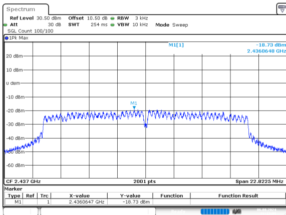
g_2437MHz
