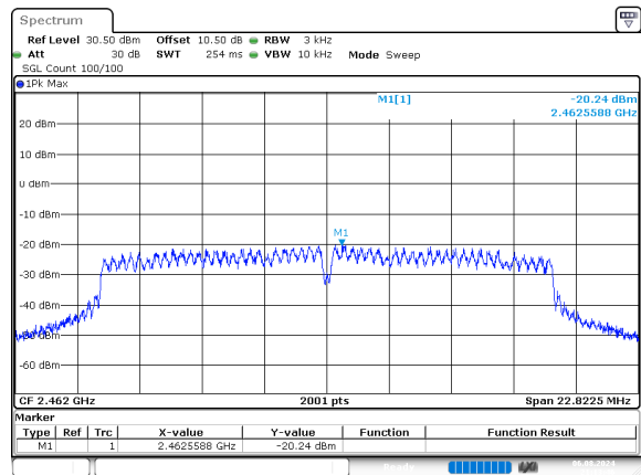
g_2462MHz
