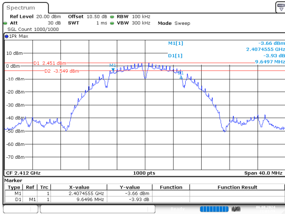
b_2412MHz
