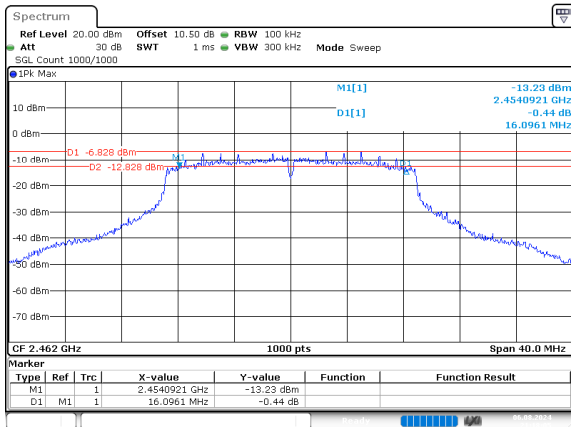
n20_2462MHz
