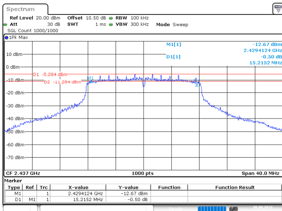
g_2437MHz
