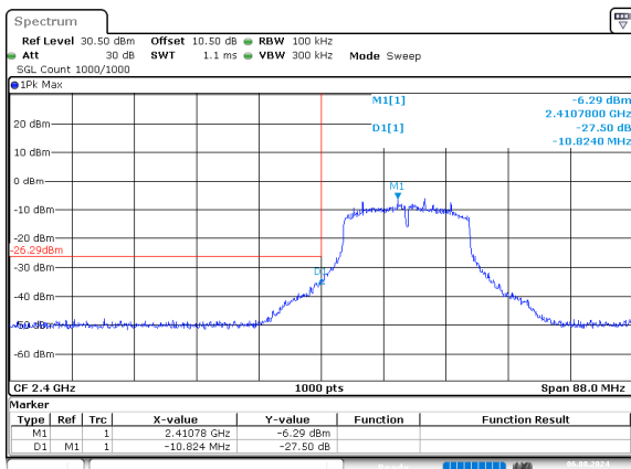
n20_2412MHz
