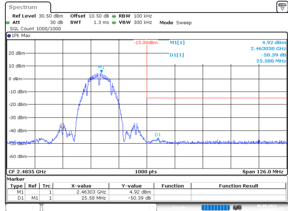
b_2462MHz
