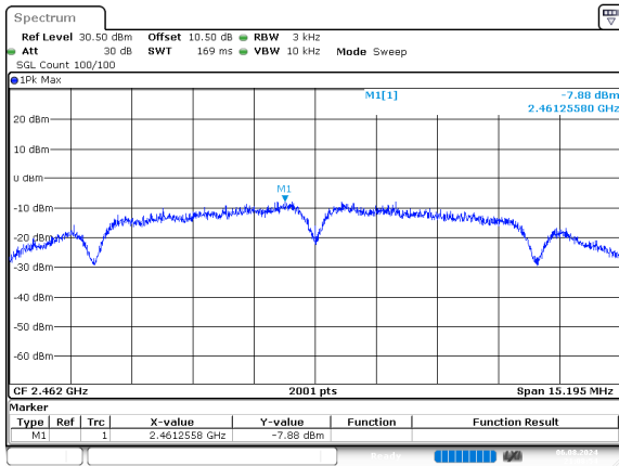
b_2462MHz
