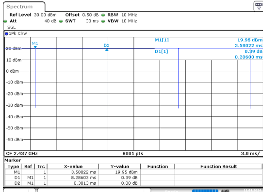
b_2437MHz_Chain 0
