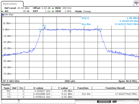
n20_2462MHz_Chain 0
