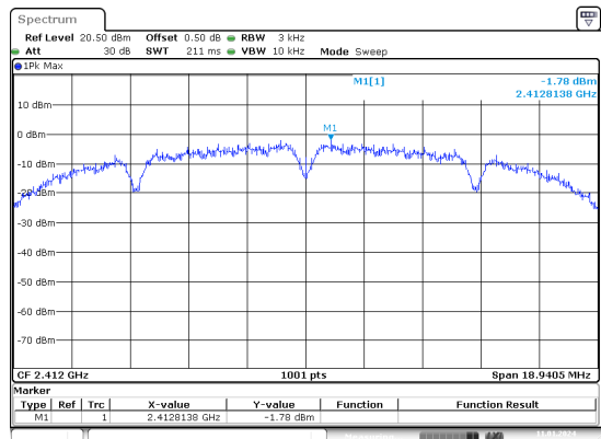
b_2412MHz_Chain 1
