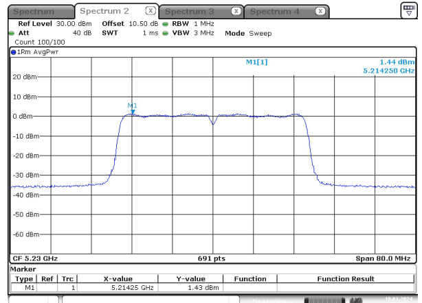
n40_5230MHz_Chain 1
