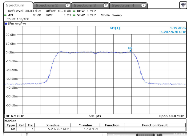
ac20_5200MHz_Chain 1
