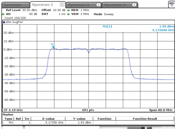
n40_5190MHz_Chain 1
