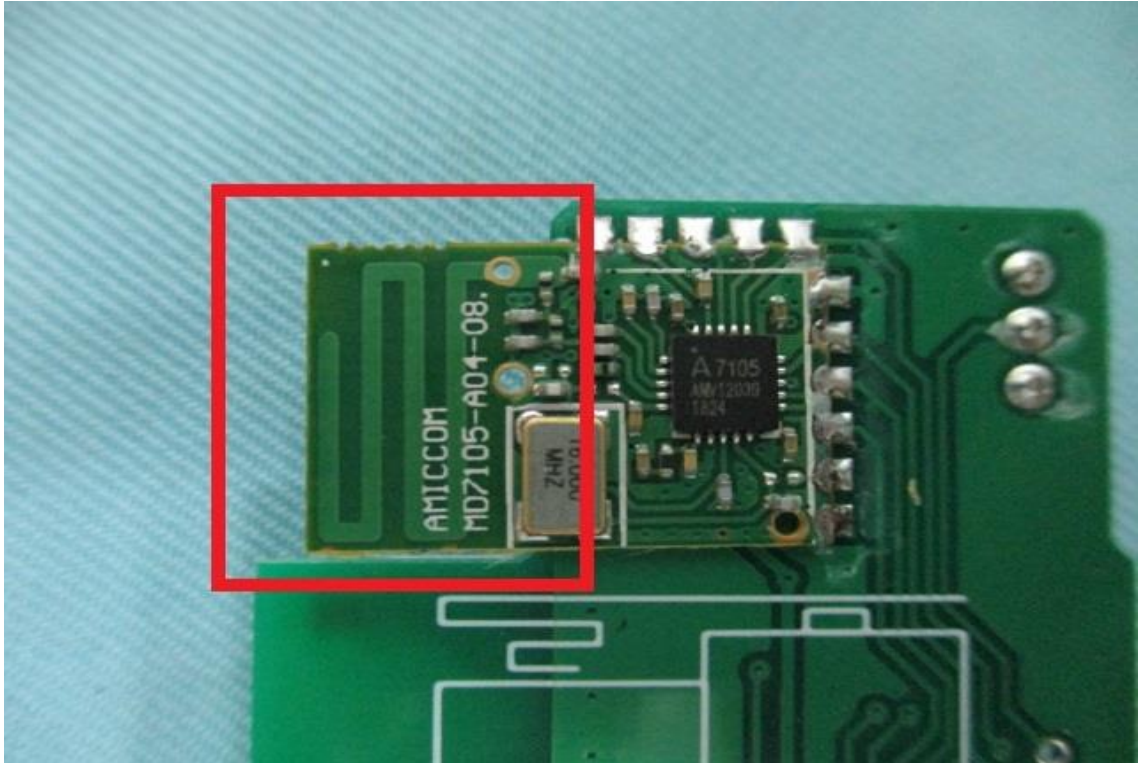
(5) PCB ANT
