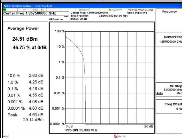
20 MHz / QPSK
