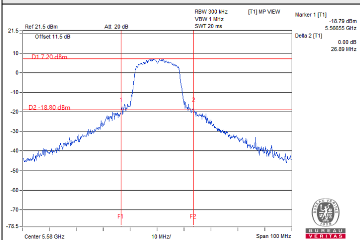
802.11a : CH 116
