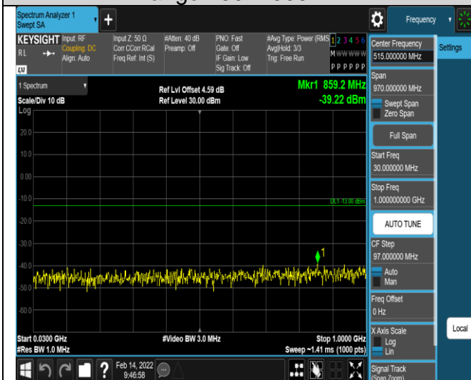
Band4-20MHz-QPSK-20300-1RB#0- Range1:30~1000MHz
