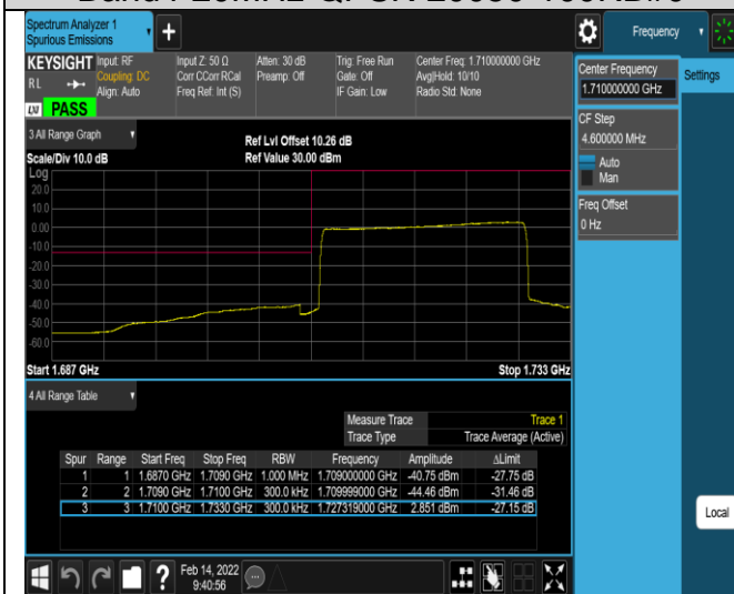
Band4-20MHz-QPSK-20300-1RB#99
