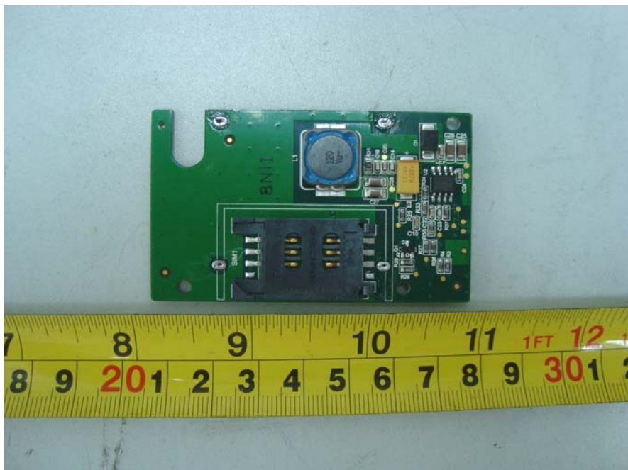
EUT – S80-GPRS-WAVECOM-V12 Board Top View
