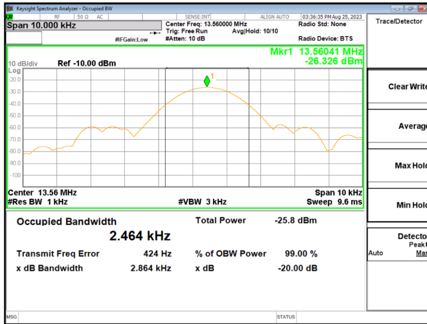
99%&20dB bandwidth
