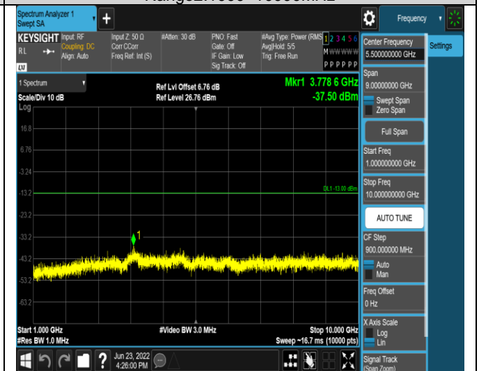
Band13-5MHz-QPSK-23255-1RB#0- Range2:1000~10000MHz
