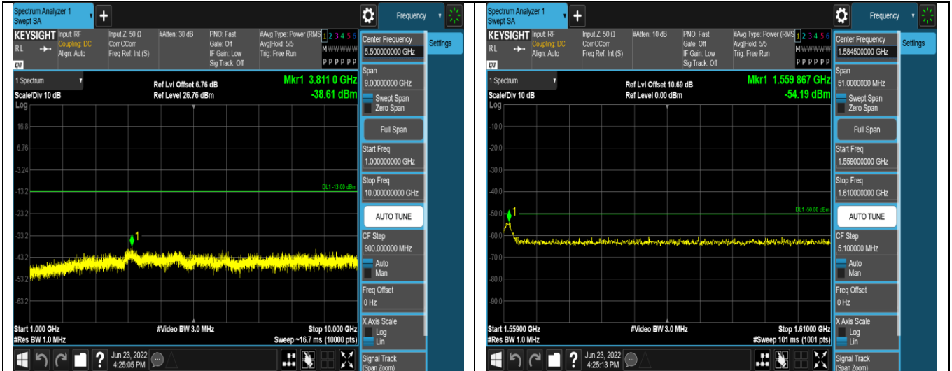
Band13-5MHz-QPSK-23255-1RB#0- Range2:1000~10000MHz
