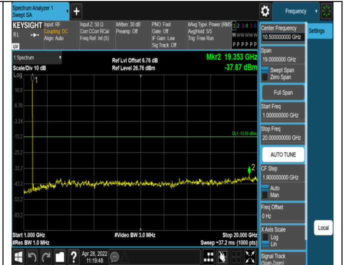
Band4-20MHz-QPSK-20175-1RB#0- Range2:1000~20000MHz
