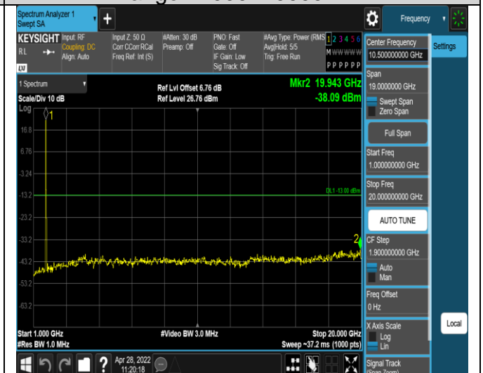
Band4-20MHz-QPSK-20300-1RB#0- Range2:1000~20000MHz
