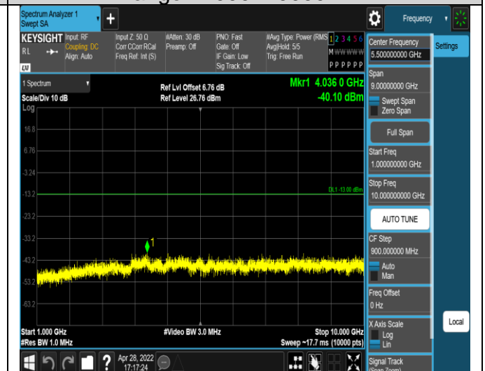
Band12-10MHz-QPSK-23130-1RB#0- Range2:1000~10000MHz
