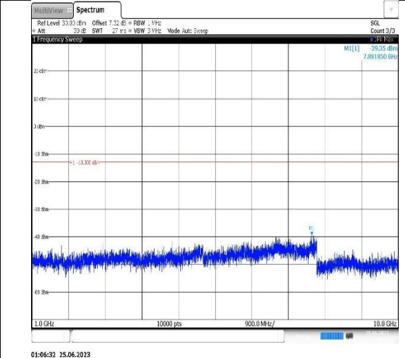
Band12-10MHz-QPSK-23130-1RB#0- Range2:1000~10000MHz
