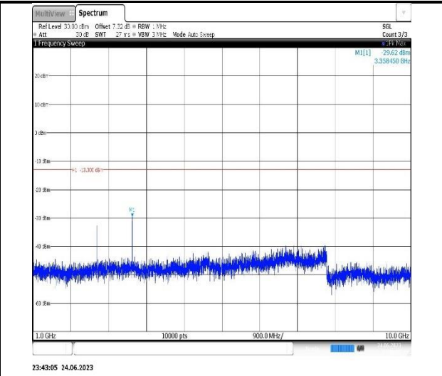
Band12-1.4MHz-QPSK-23017-1RB#0-Range2:1000~10000MHz
