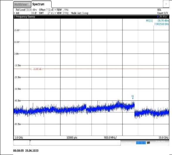
Band12-5MHz-QPSK-23155-1RB#0-Range2:1000~10000MHz
